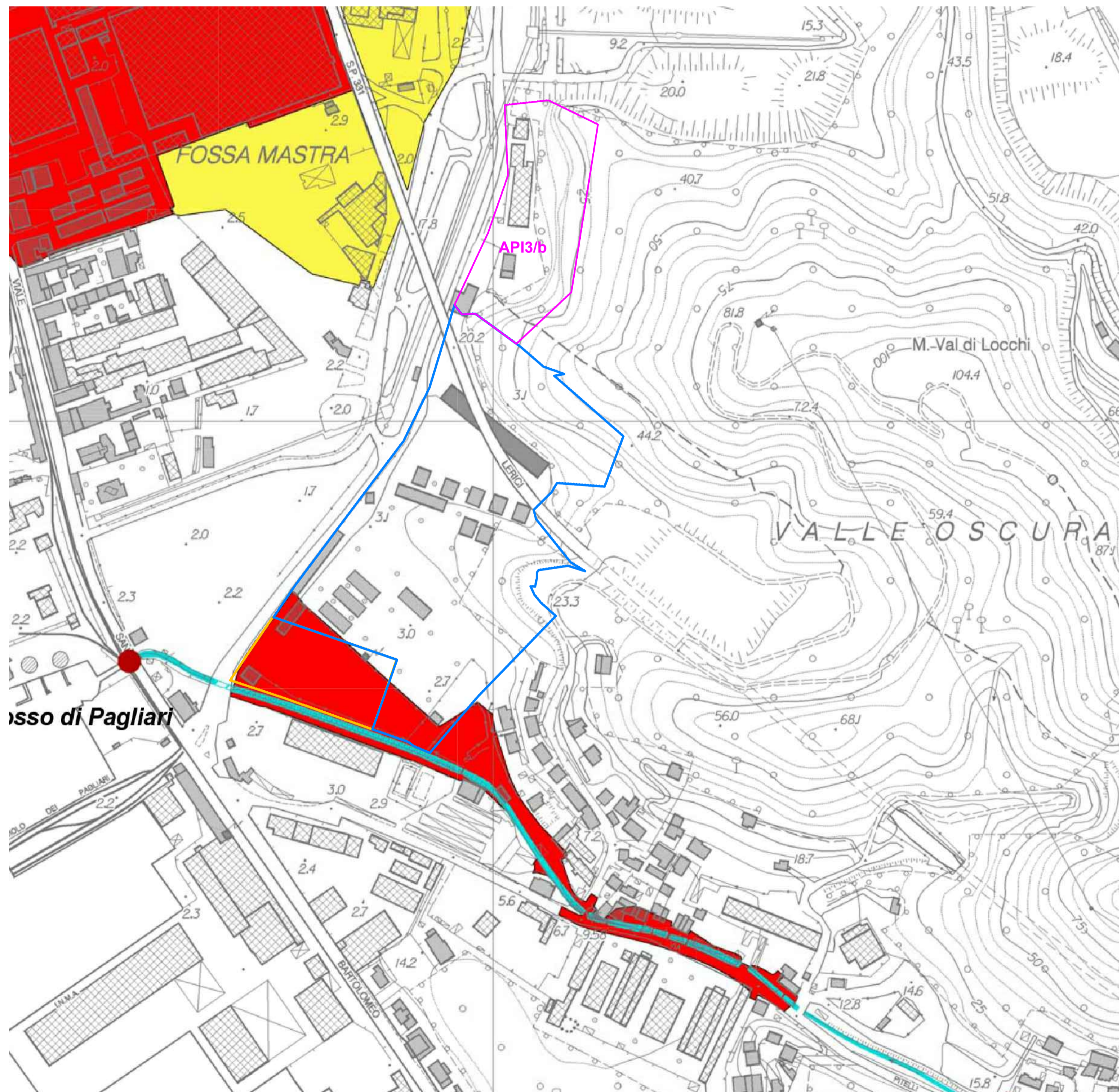
Estratto di mappa di inondabilità con sovrapposizione lotti di intervento scala 1/2000
