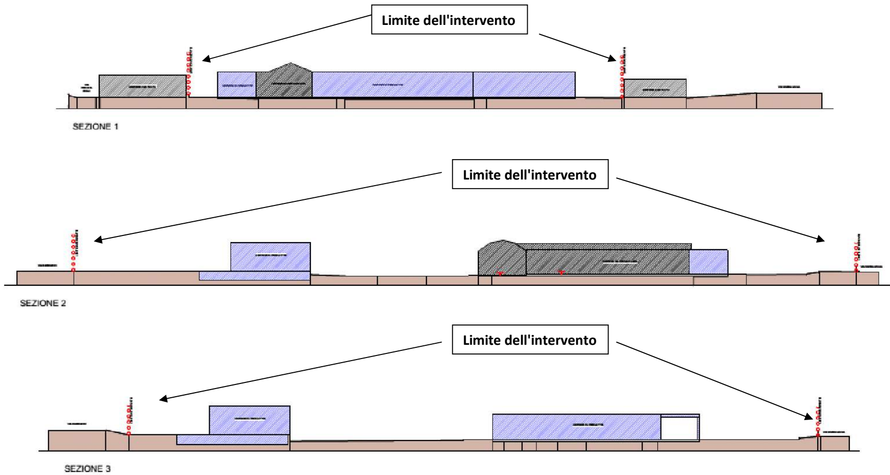
Tav 2 - sezioni schematiche
